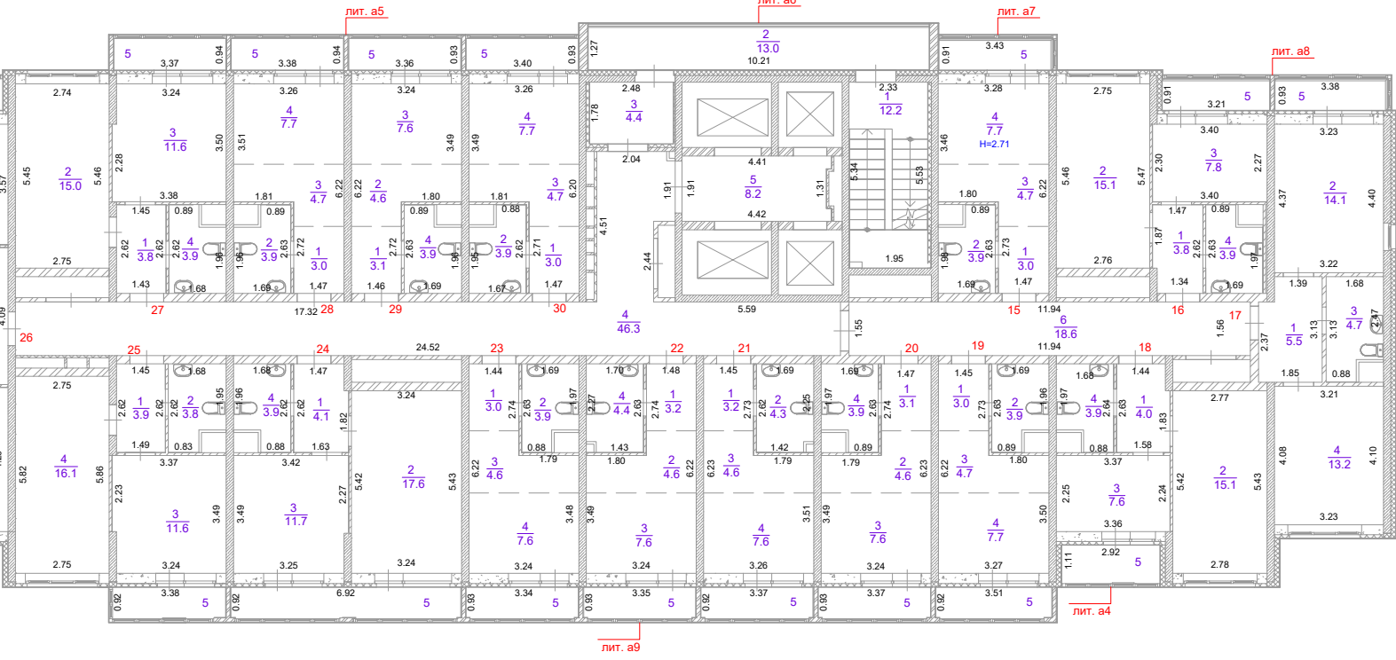
План 2 этажа Секция 1.1
