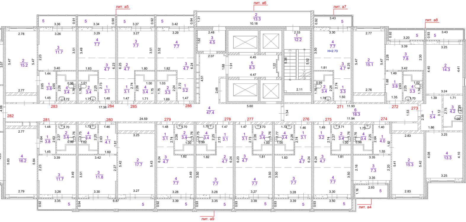
План 18 этажа Секция 1.1
