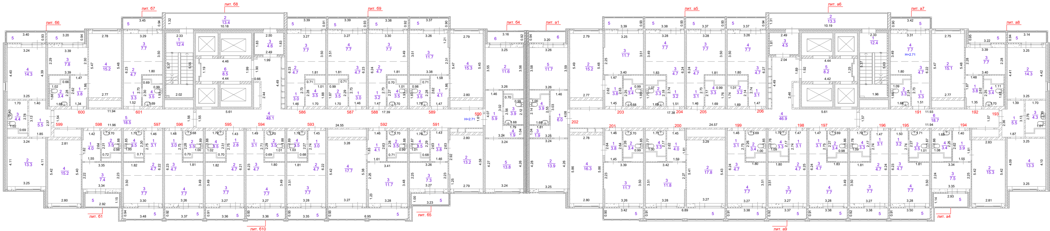
План 13 этажа Секция 1.2
