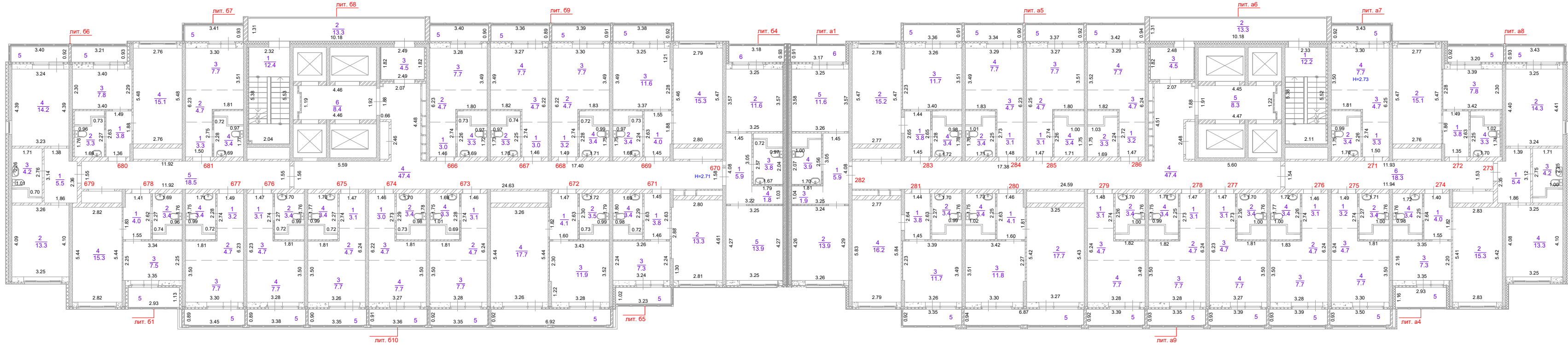
План 18 этажа Секция 1.2
